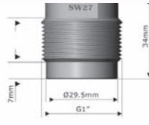
Schwinggabeladapter 1* HEM-10
