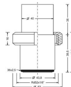
Typ B Nutmutteradapter Ø44mm
