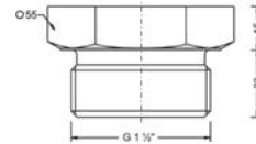
Typ 7 G 1 1/2" ISO 228-1 – frontbündig
